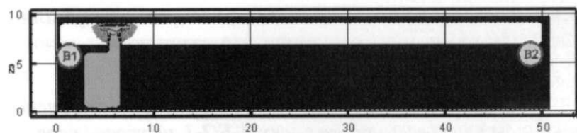
Рис. 4. Поля оптической плотности дыма ( Hn/m ) в горизонтальном сечении на высоте 1,7 м от уровня пола в момент времени 80 с
