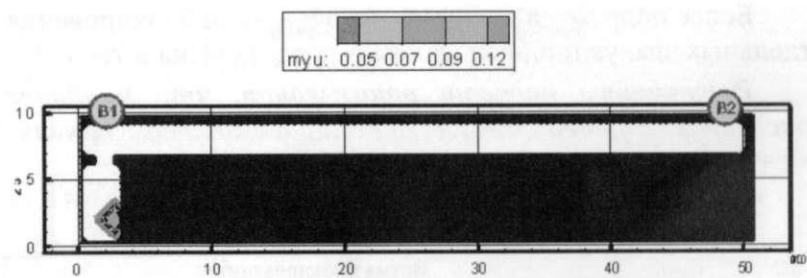
Рис. 13. Оптическая плотность дыма (Нп/м) в горизонтальном сечении на высоте 1,7 м от уровня пола в момент времени 40 с
