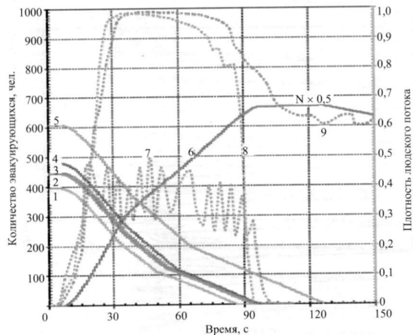
Рис. 38. Динамика эвакуации людей с 16-го и 11-го этажей.
