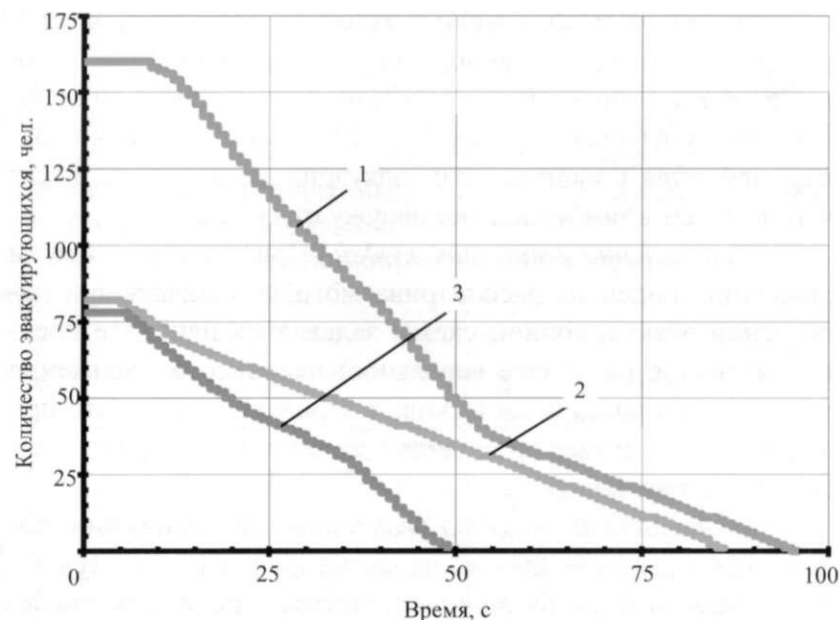
Рис. 27. Динамика эвакуации людей из жилого здания:
