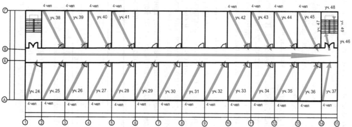
Рис. 26. Расчетная схема эвакуации для сценария № 2
