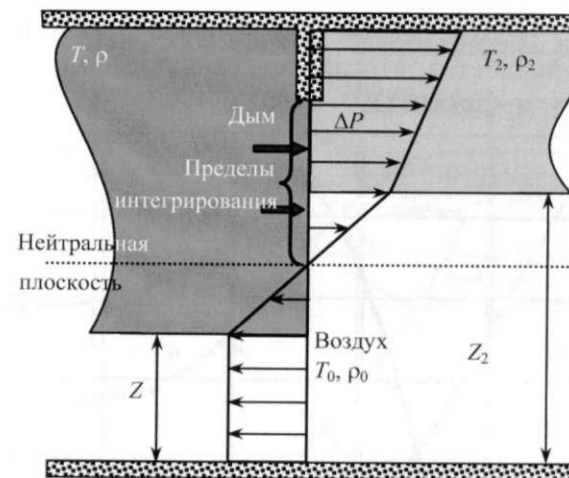
Рис. 31. Массопотоки через проем
