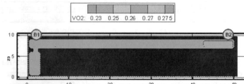
Рис. 23. Концентрация O 2 (кг/м 3 ) в горизонтальном сечении на высоте 1,7 м от уровня пола в момент времени 340 с
