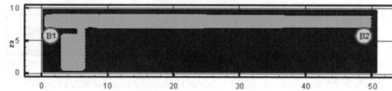
Рис. 9. Поля температуры ( K ) в горизонтальном сечении на высоте 1,7 м от уровня пола в момент времени 360 с
