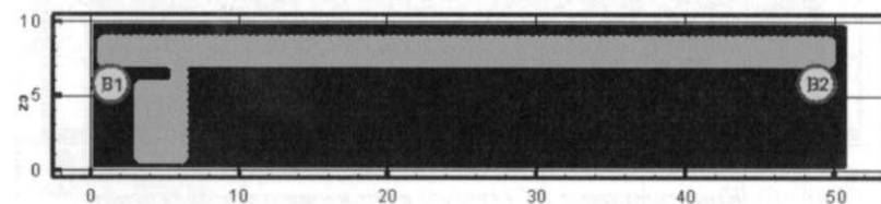
Рис. 7. Поля оптической плотности дыма ( Hn/m ) в горизонтальном сечении на высоте 1,7 м от уровня пола в момент времени 360 с
