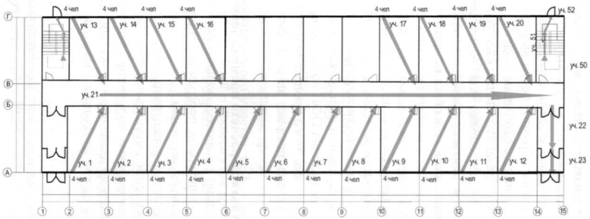
Рис. 25. Расчетная схема эвакуации для сценария № 1
