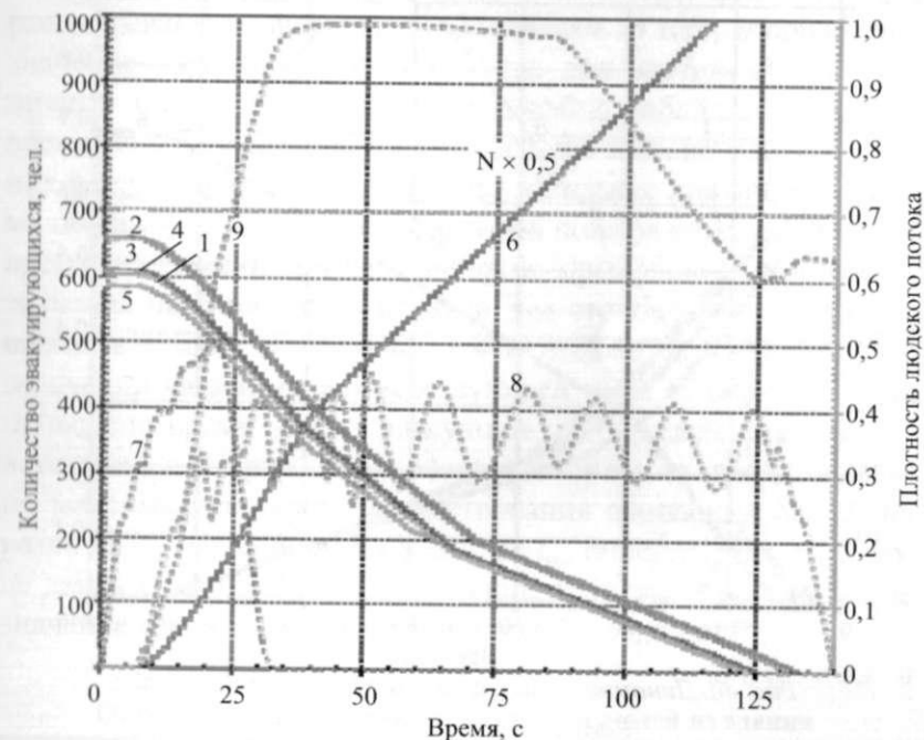
Рис. 39. Динамика эвакуации людей с 10-го и 6-го этажей.
