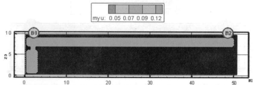
Рис. 17. Оптическая плотность дыма (Нп/м) в горизонтальном сечении на высоте 1,7 м от уровня пола в момент времени 340 с
