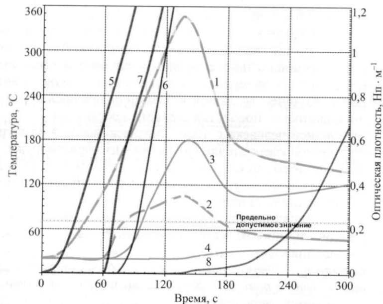
Рис. 35. Динамика температуры (1÷4) и оптической плотности дыма (5÷8) при пожаре в помещении офиса (сценарий 2).
