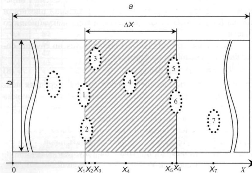
Рис. 24. Координатная схема размещения людей на путях эвакуации
