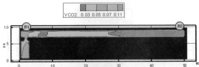
Рис. 20. Концентрация CO 2 (кг/м 3 ) в горизонтальном сечении на высоте 1,7 м от уровня пола в момент времени 340 с
