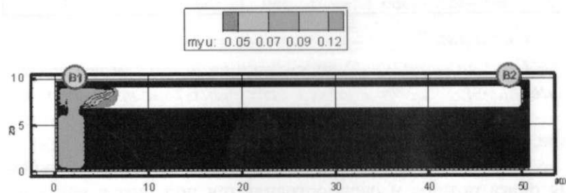
Рис. 14. Оптическая плотность дыма (Нп/м) в горизонтальном сечении на высоте 1,7 м от уровня пола в момент времени 80 с
