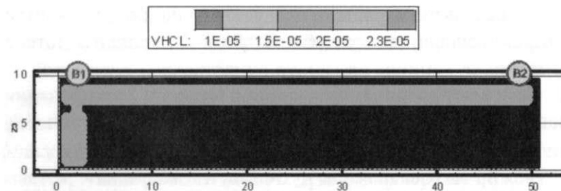
Рис. 22. Концентрация HCl (кг/м 3 ) в горизонтальном сечении на высоте 1,7 м от уровня пола в момент времени 340 с
