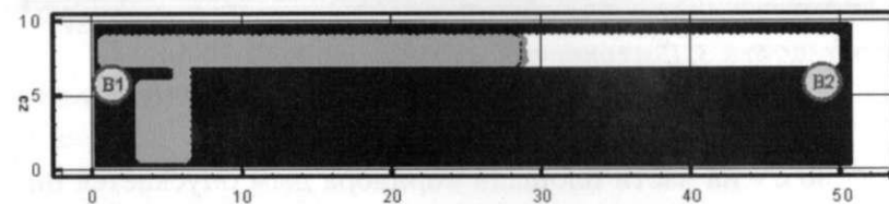
Рис. 6. Поля оптической плотности дыма ( Hn/m ) в горизонтальном сечении на высоте 1,7 м от уровня пола в момент времени 300 с
