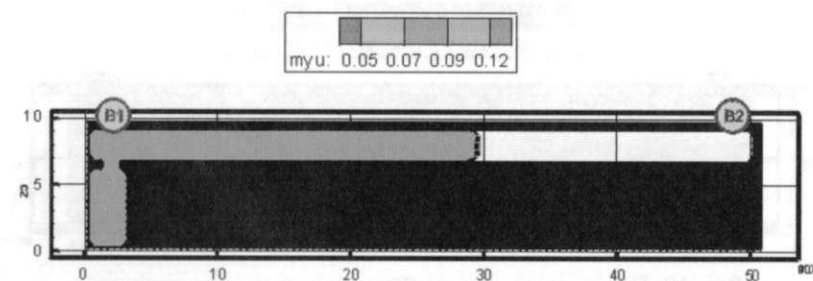
Рис. 16. Оптическая плотность дыма (Нп/м) в горизонтальном сечении на высоте 1,7 м от уровня пола в момент времени 280 с
