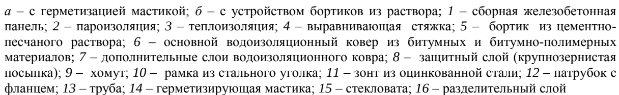
Рисунок Ж.5 – Пропуск трубы через покрытие с традиционной кровлей
