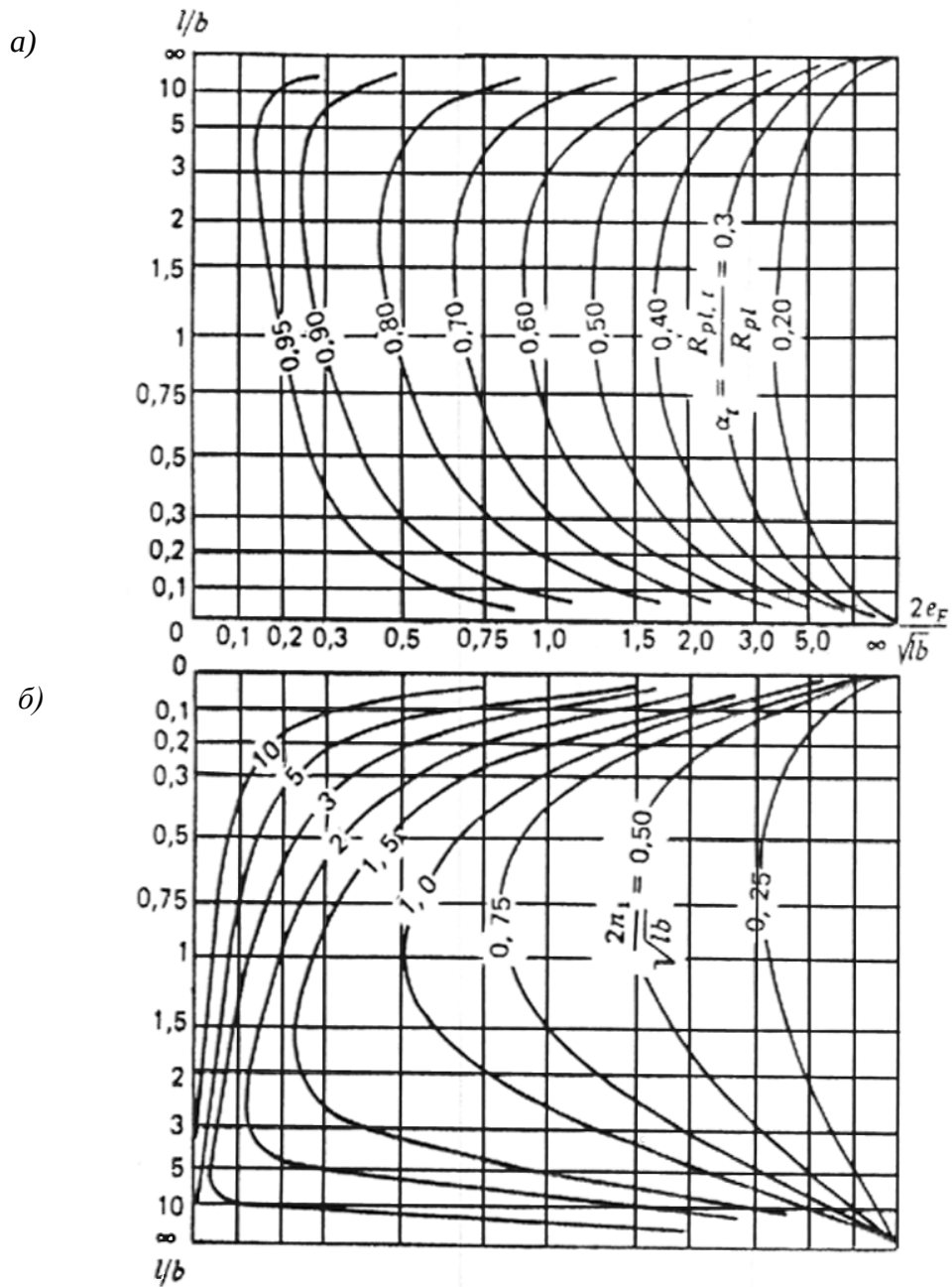
Рисунок Д.2 – Графики для определения коэффициента \alpha_t (a) и координаты центра поворота n_1 (б)
