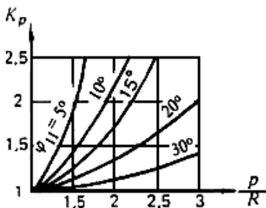
Рисунок Л.1 – График для определения коэффициента K_p
