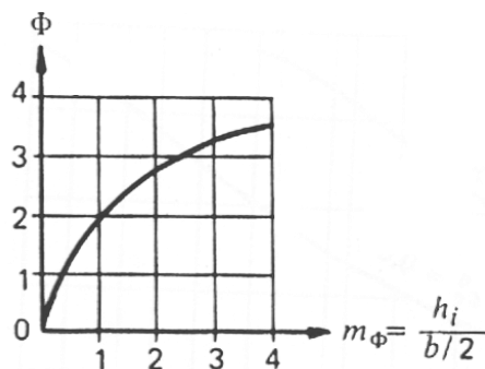
Рисунок Н.2 – График для определения коэффициента \Phi
