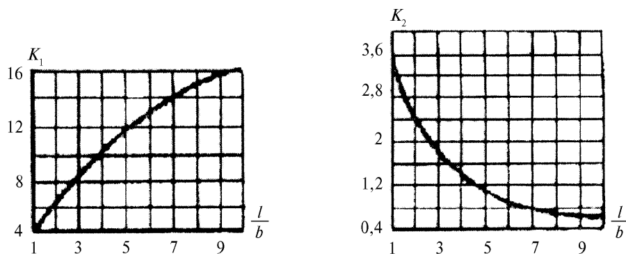
Рисунок 1 – Графики для определения коэффициентов K_1 и K_2
