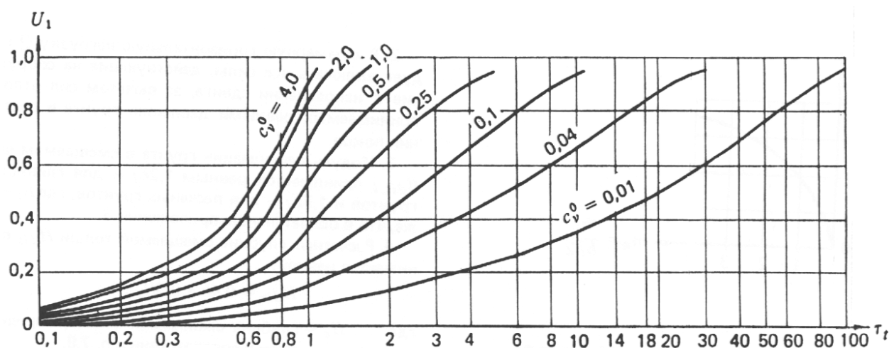
Рисунок М.1 – График зависимости степени консолидации
