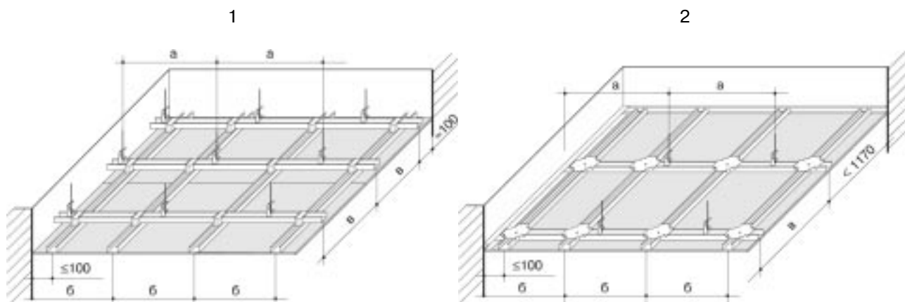
Рисунок 13 — Конструкции подвесных потолков 1 — конструкция двухуровневого потолка; 2 — конструкция одноуровневого потолка; a — расстояние между подвесами, b — расстояние между несущими профилями, v — расстояние между основными профилями
