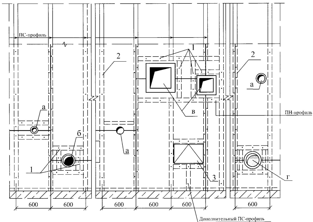
Рисунок 5 — Схема размещения трубопроводов диаметром не более 60 мм (а), технологических трубопроводов — не менее 60 мм (б), воздуховодов (в) и трубопроводов водоснабжения и отопления (г)
