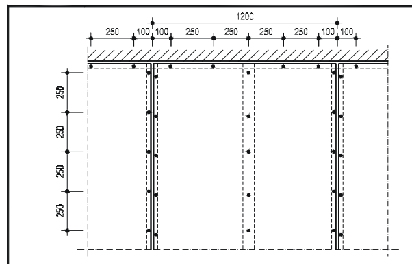
Рисунок 18 — Крепление гипсоволокнистых листов к каркасу
