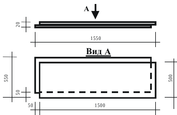
Рисунок 14 — Элемент сборного основания пола
