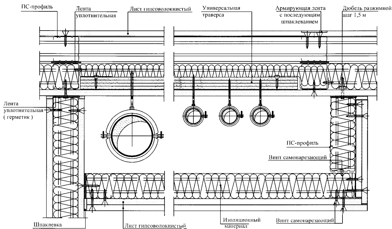
Рисунок 11 — Конструктивные решения ограждения коммуникационных шахт у несущей стены (а) и у перегородки (б)
