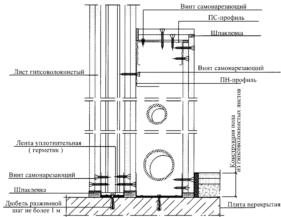
Рисунок 10 — Конструктивное решение обрамления трубопроводов, размещенных вдоль капитальной стены (а), перегородки (б)
