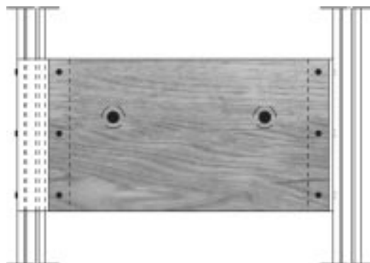
Рисунок 19 — Универсальная деревянная траверса
