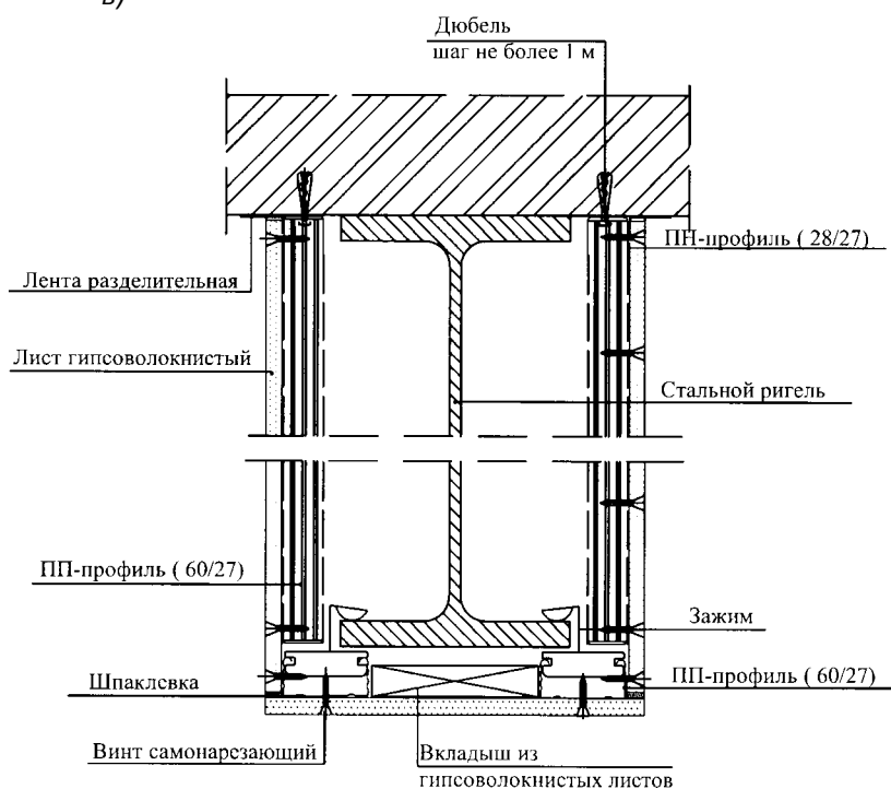
Рисунок 15 — Конструктивное решение огнезащиты стальных балок гипсоволокнистыми листами
