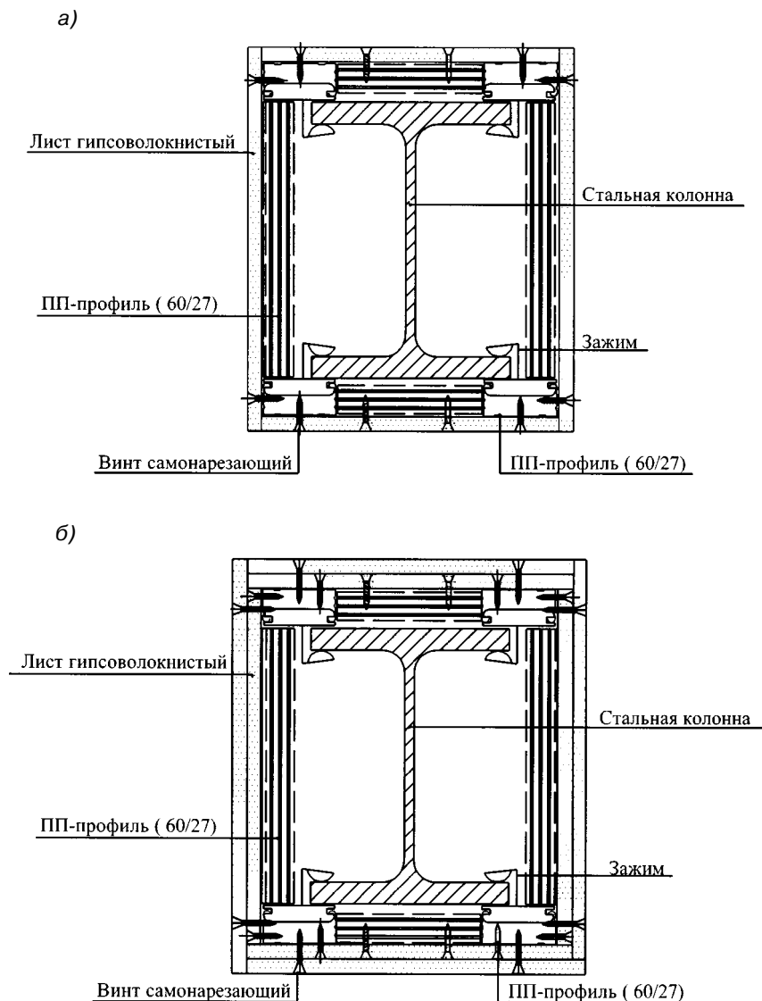
Рисунок 17 — Конструктивное решение огнезащиты стальных колонн гипсоволокнистыми листами
