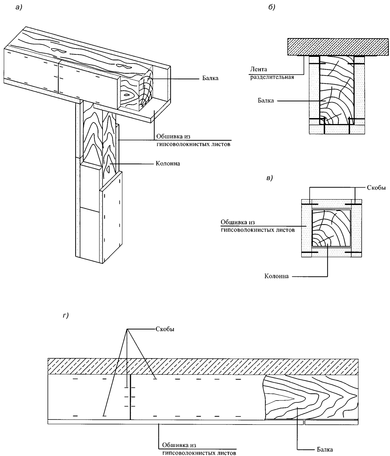
Рисунок 16 — Общий вид (а), конструктивное решение огнезащиты деревянной балки (б, г) и колонны (в)
